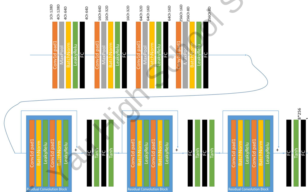
图6 BPCNN网络结构图
