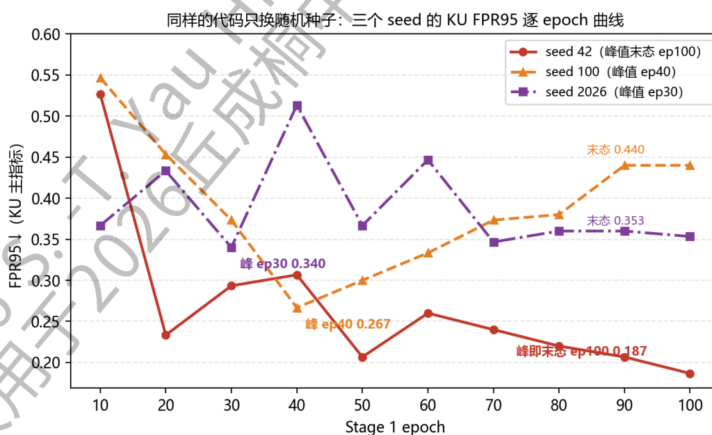
图 5 三个训练随机种子下的跨域 FPR95 演进轨迹。seed 42 在第 100 轮达最优工作点, 而 seed 100 与 2026 的极值点分别提前至 40 与 30 轮且后续发生退化。
