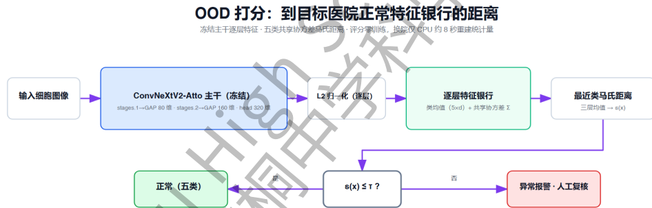
图 2 轻量特征提取、统计评分与报警工作流。新细胞切图经冻结骨干网络映射至特征空间，计算其到五个正常类中心的共享协方差马氏距离；最小距离超阈即触发报警。
