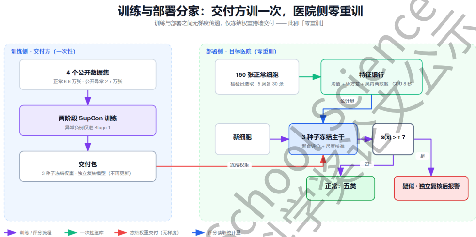
图 1 系统总体架构与两阶段跨域部署 workflow。左（模型研发侧）：基于四个公开多源数据集构建通用特征空间，输出后冻结权重；右（基层部署侧）：目标医院检验员仅需选取少量正常细胞在普通 CPU 上快速生成本地特征库，待检样本经多级聚合评分与轻量二级复核后触发分流。
