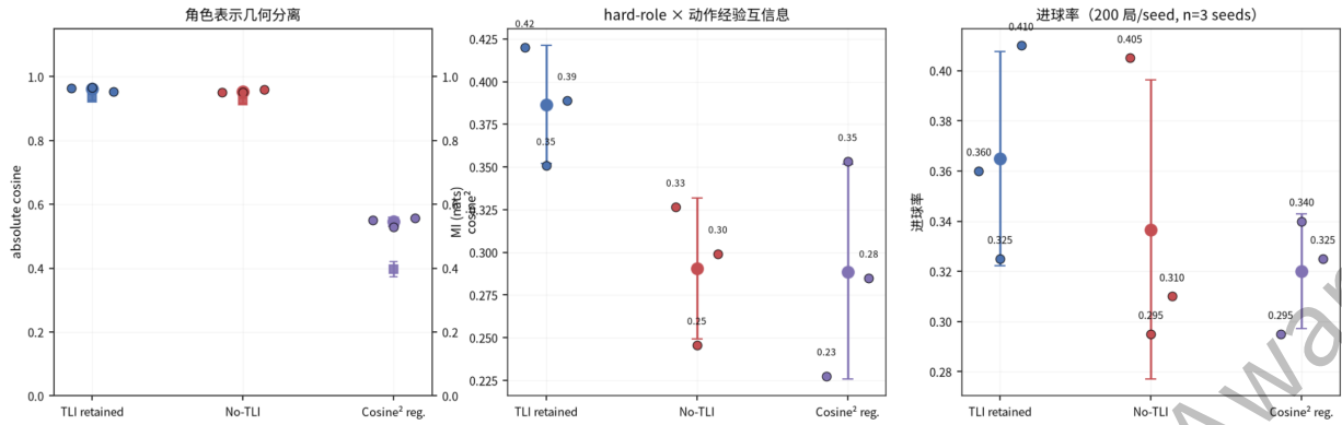
图3 角色几何变化、实际行为关联与任务表现的对应关系。每个小点表示一个训练种子，误差条为三种子均值与标准差。
