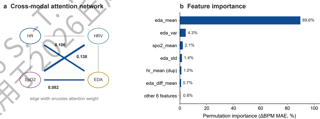
图 14 注意力关系与特征重要性（实测值）
