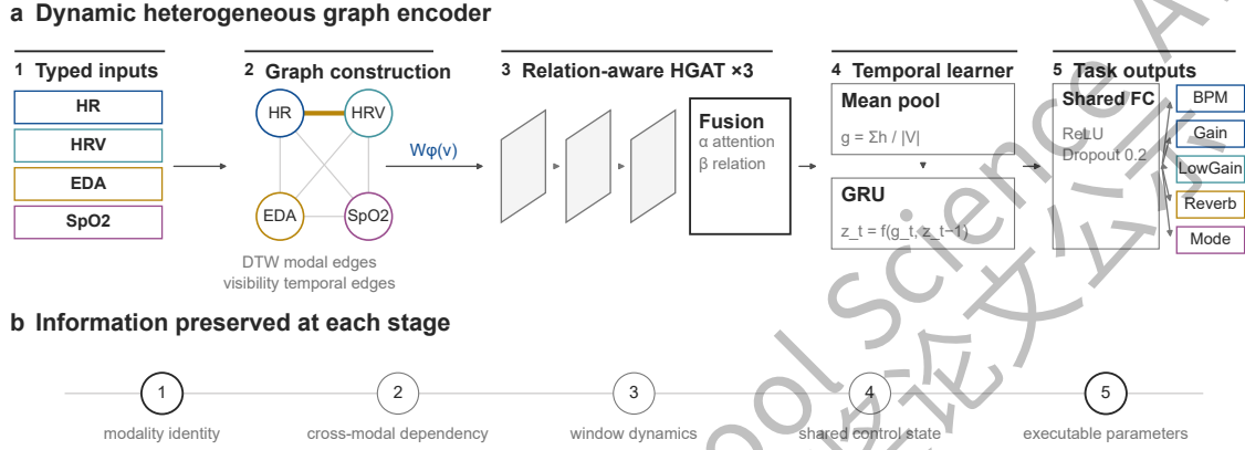
图 4 DHGNN 核心架构。(a) 动态异构图编码器的五个计算阶段。(b) 各阶段保留的信息语义。
