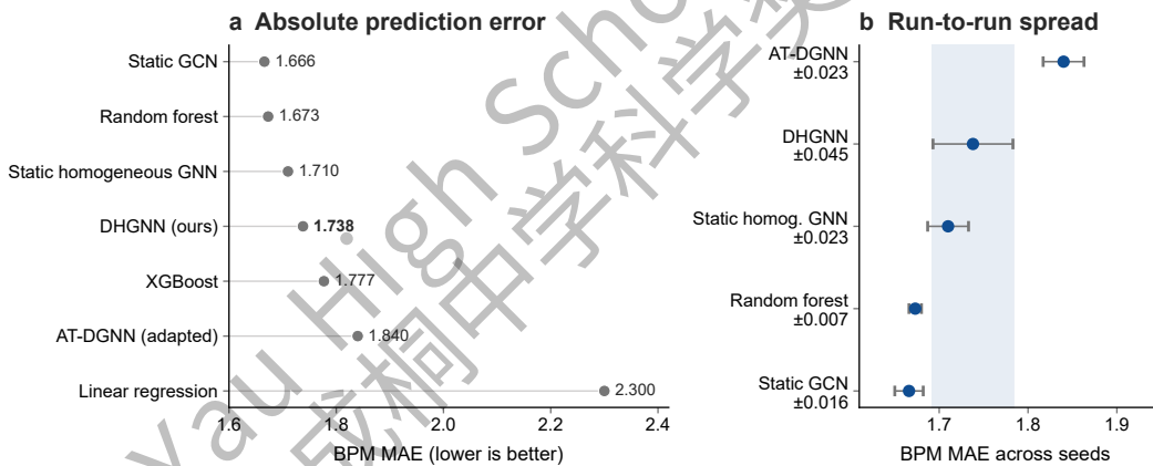
图 12 各模型 BPM 预测误差对比（实测值）
