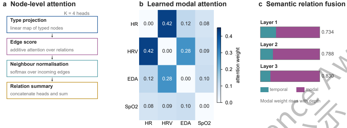
图 6 异构图注意力机制。(a) 节点级注意力计算：类型投影 h'_v = W_{\phi(v)}x_v 、边得分 e_{st}^{r,k} = a^T[W_r h_s \| W_r h_t] 、邻居归一化 \alpha_{st}^{r,k} = \text{softmax}_s(e_{st}^{r,k}) 、关系汇总 h_v^r = \sum_s \alpha_{st}^{r,k} W_r^k h_s 。(b) 跨模态注意力矩阵。(c) 语义关系融合，融合节点状态为 h_v^{(l)} = \sum_r \beta_r h_v^{(r,l)} + h_v^{(l-1)} 。
