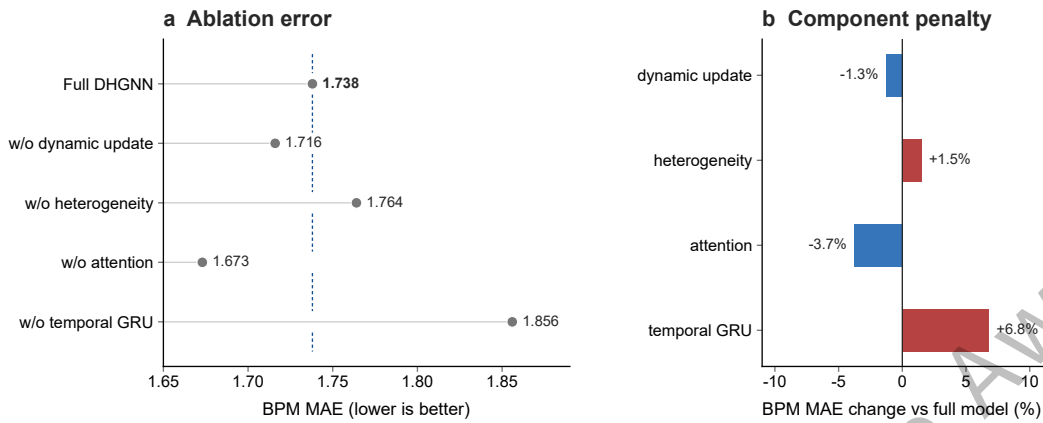
图 13 DHGNN 各模块消融后的 BPM 预测误差 (实测值)
