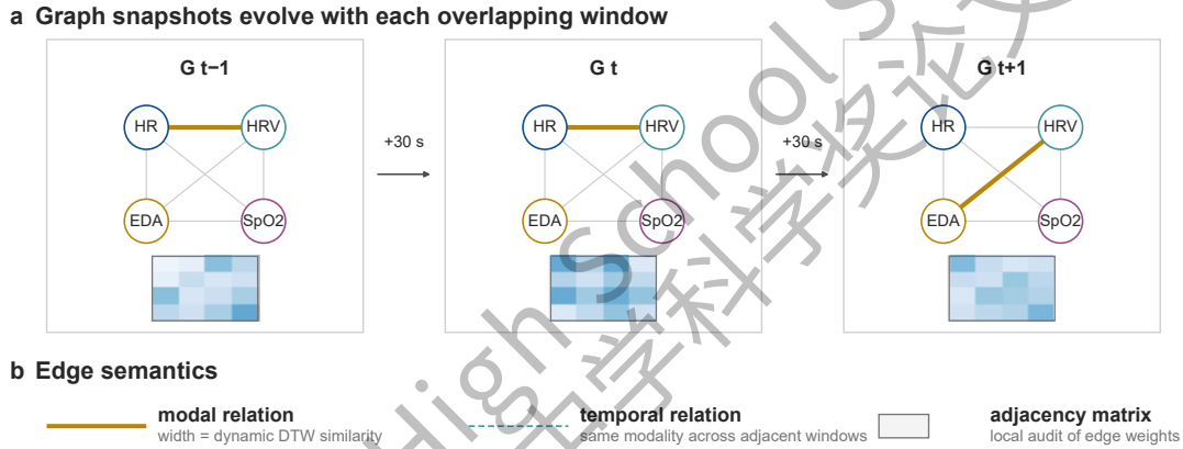
图 5 滑动窗口推进过程中的动态异构图演化。(a) 连续图快照与邻接矩阵。(b) 模态边、时序边与矩阵编码的图例说明。
