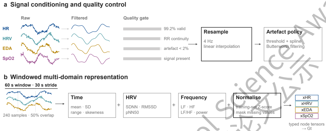
图 2 多模态生理信号的数据准备与特征工程。(a) 信号调理与质量控制。(b) 滑动窗口、多域特征及类型化节点张量的形成。
