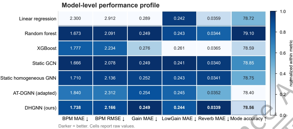
图 11 各模型多任务预测性能矩阵（实测值）
