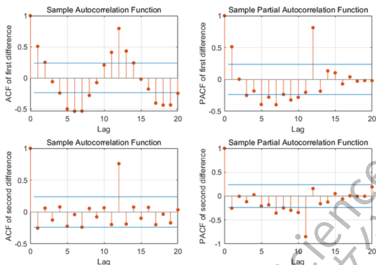
图 13 ACF 与 PACF 图
