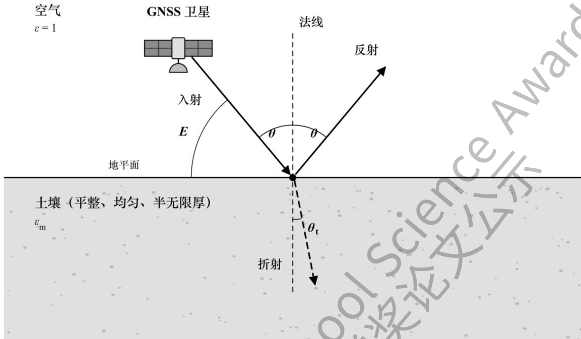
图 2.2 空气与土壤界面几何关系
