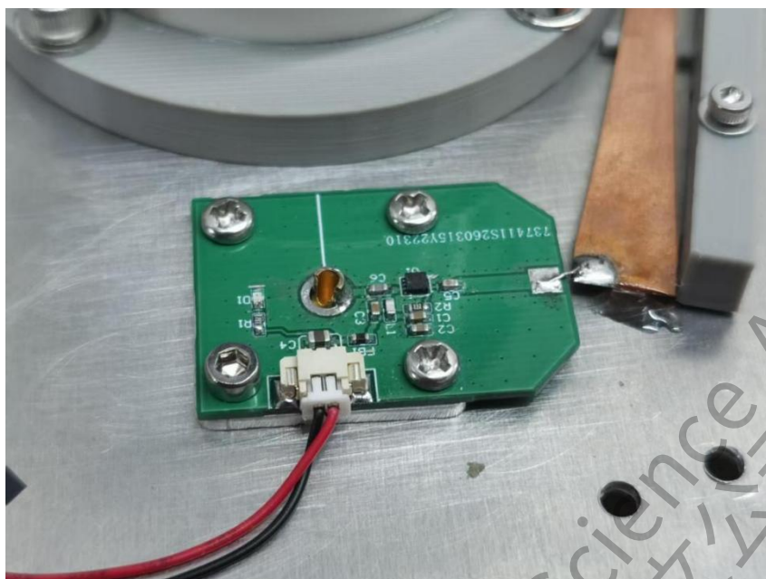
图 3.14 QPL9547 低噪声放大电路实物
