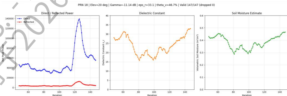
图 5.14 半主动式反演结果（高湿土，PRN 18， \Gamma = -11.14 dB， \theta_v = 46.7\% ）
