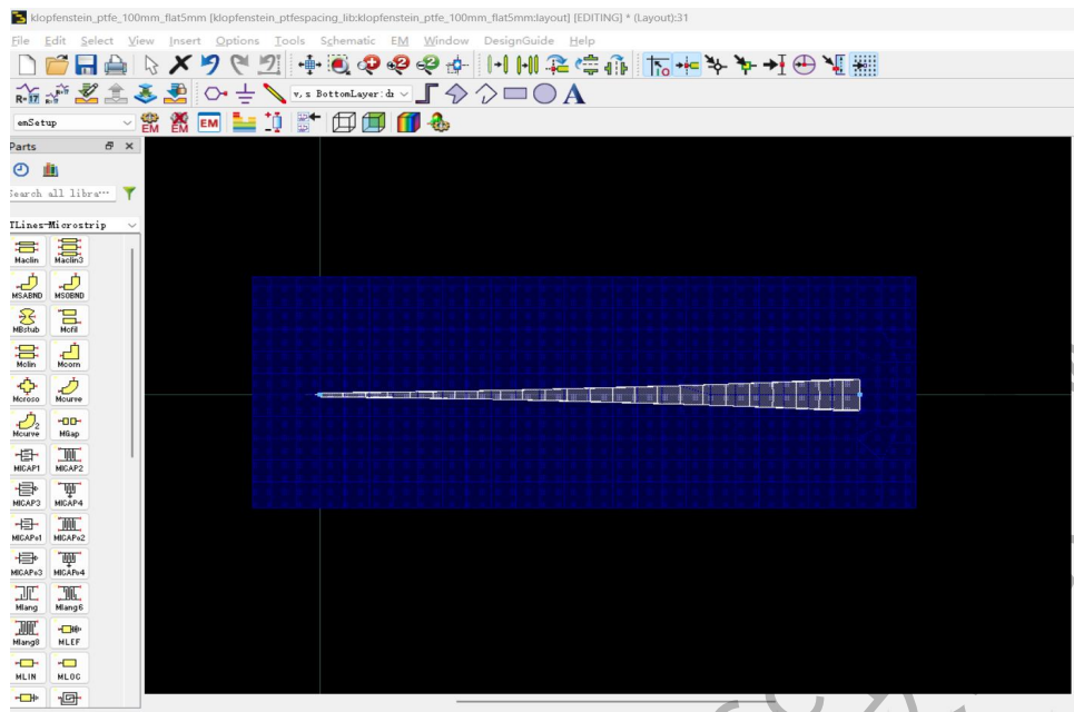
(b) 导入 dxf 文件的阻抗匹配渐变线模型
