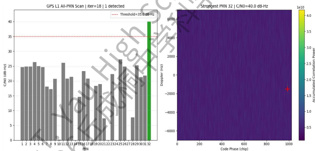
图 5.9 第二组全 PRN 搜索及 PRN 32 二维相关结果
