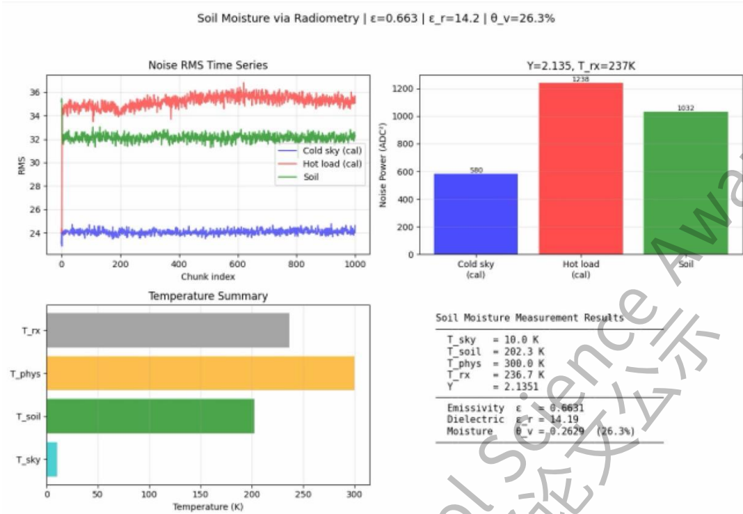
图 4.17 土壤湿度反演结果 (测量 D, Y=2.14)
