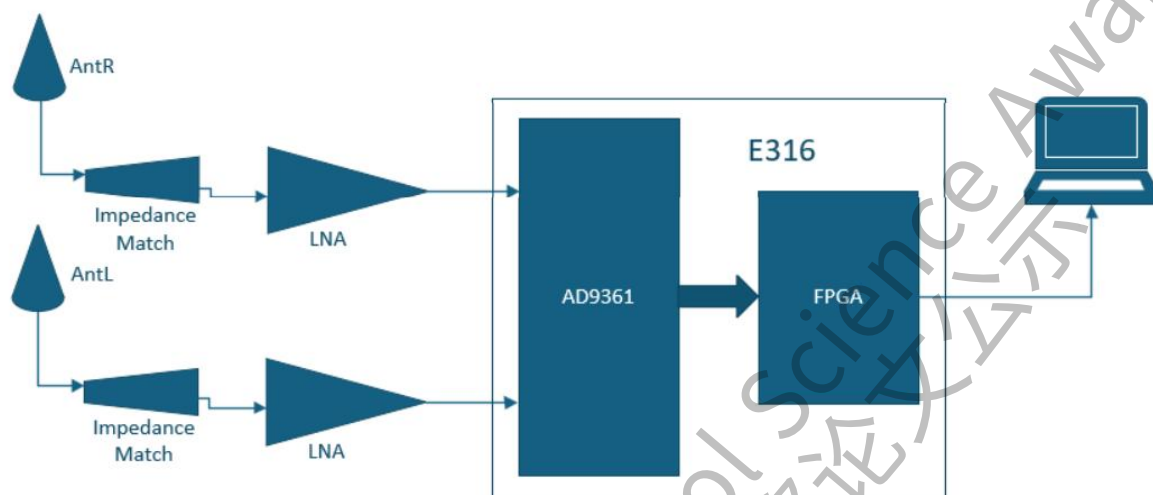
图 4.3 系统连接方式示意图
