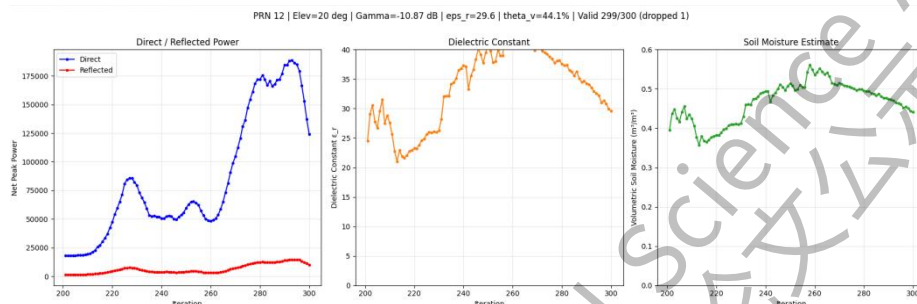
图 5.16 半主动式反演结果（高湿土，PRN 12， \Gamma = -10.87 dB， \theta_v = 44.1\% ）
