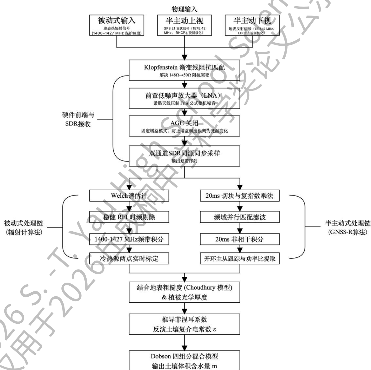
图 1.1 全文结构图
