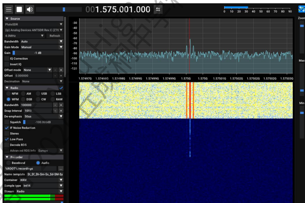
图 4.6 SDRPP 接收信号（红线有三条的原因是载波频率用 1KHz 的信号进行了 AM 调制）
