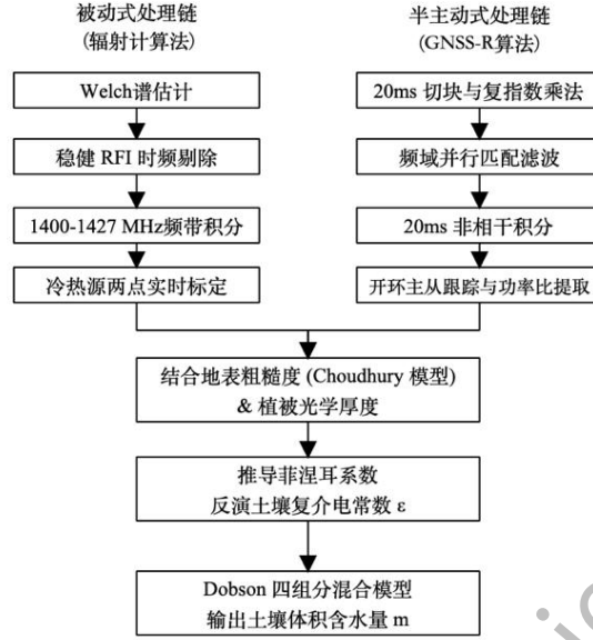
图 3.1 双链路系统结构
