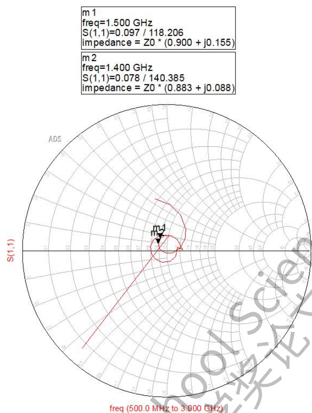
(b) 输入阻抗 Smith 圆图
