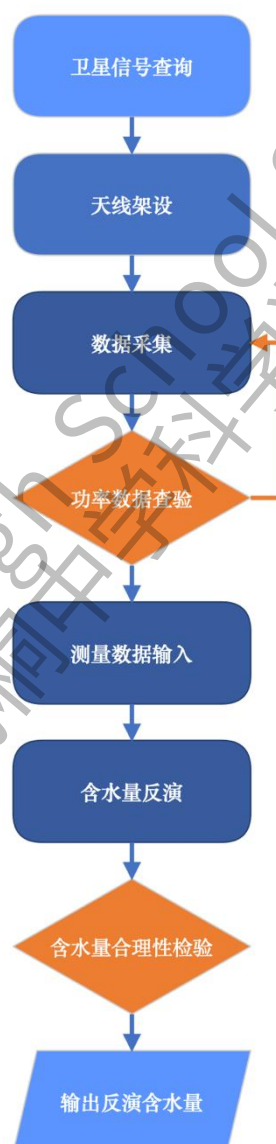
图 5.4 半主动式实验流程示意图
