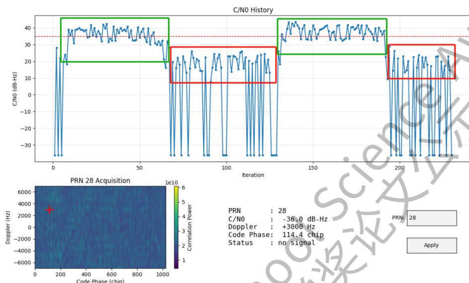
图 5.10 PRN28 连续捕获稳定性结果
