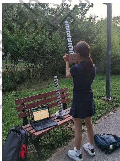
图 4.8 冷参考观测(室外开阔环境下天线指向高仰角天空)
