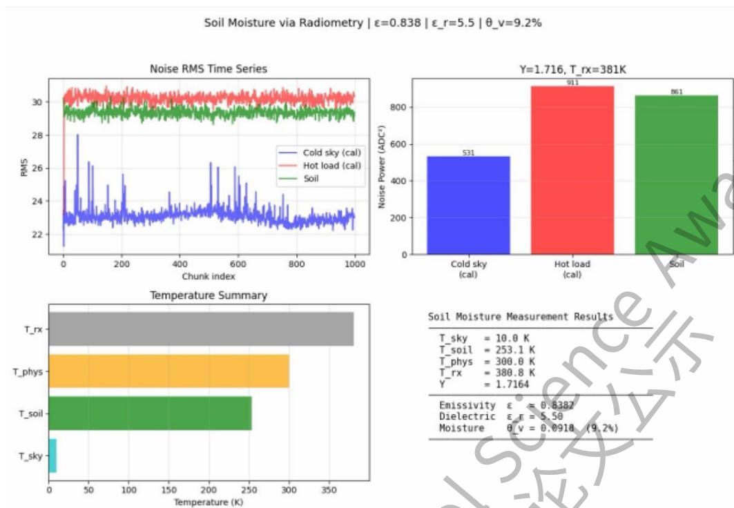
图 4.15 土壤湿度反演结果 (测量 B, Y=1.72 )
