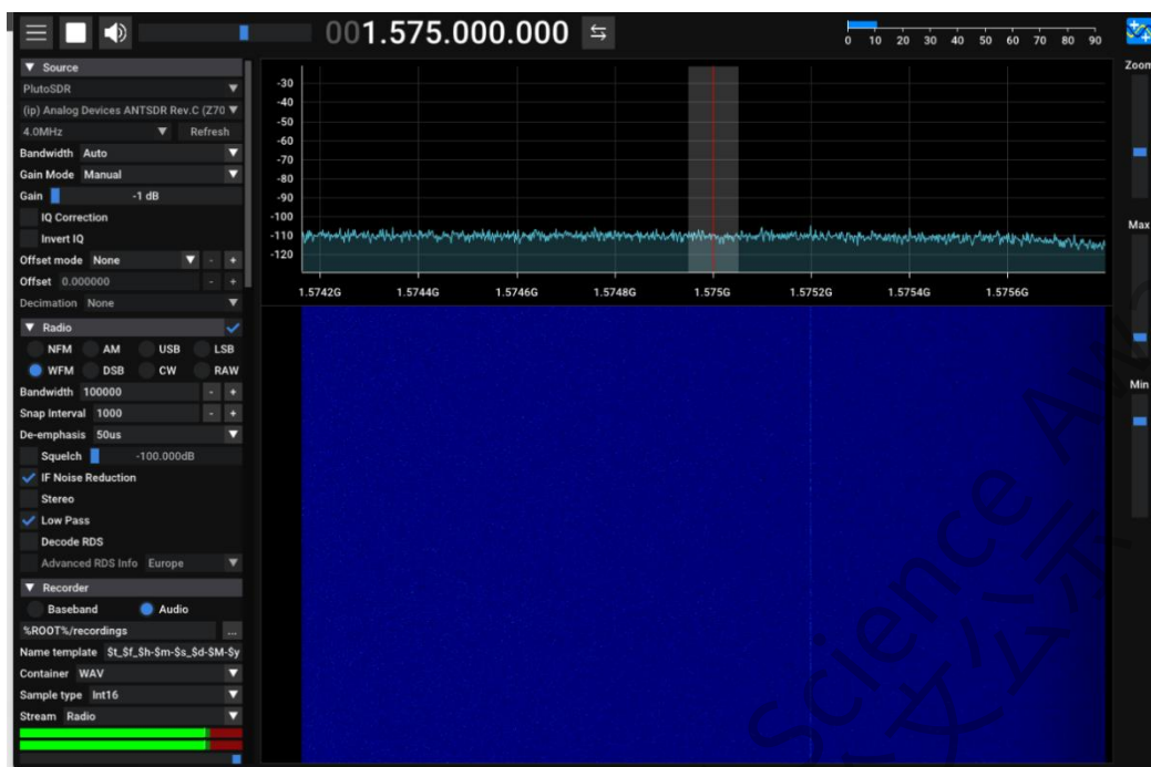
图 4.5 SDRPP 连接 E316，右侧暗线可能是内部信号泄漏
