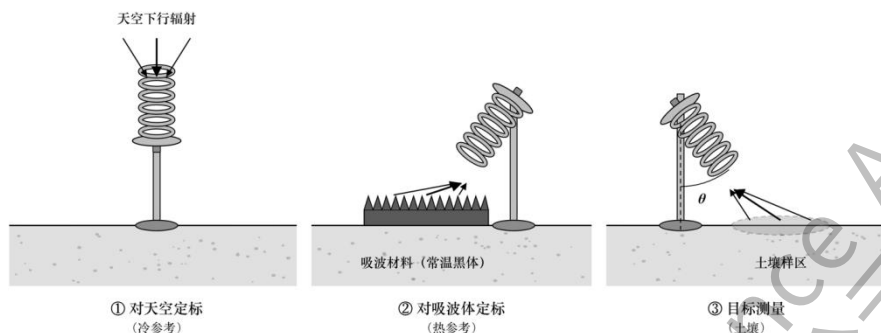
图 4.1 被动式测量示意图
