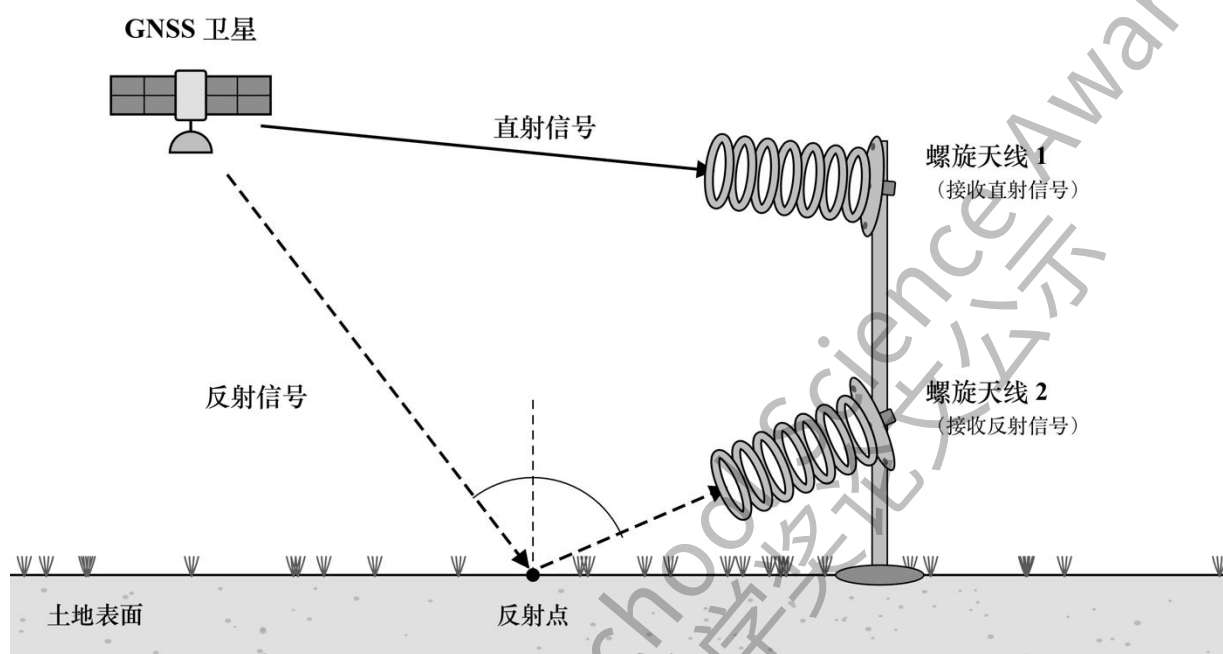
图 5.1 半主动式测量示意图
