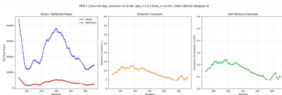
图 5.15 半主动式反演结果（干燥砂质土，PRN 5， \Gamma = -8.10 dB， \theta_v = 10.0\% ）
