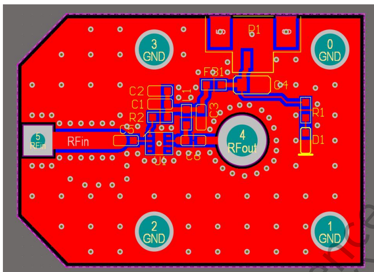
(b) PCB 版图
