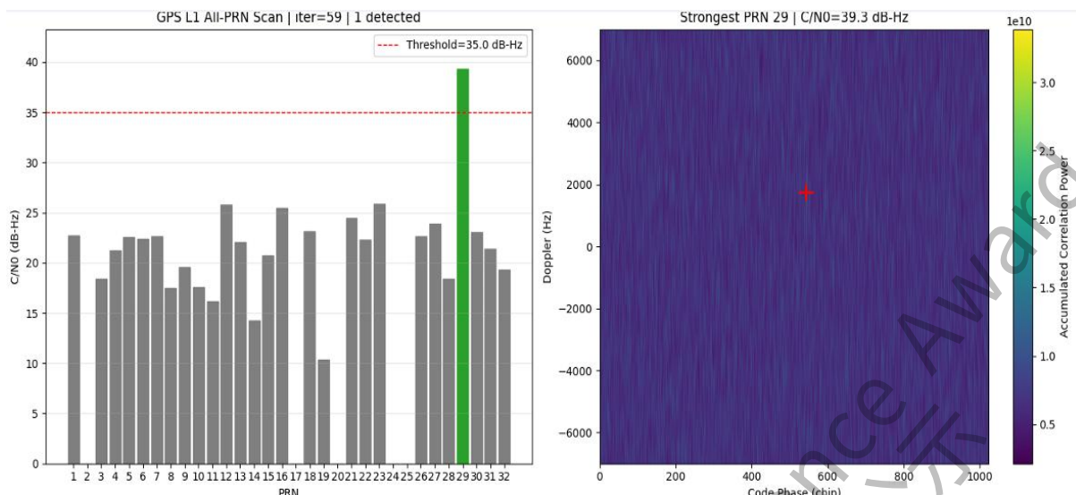
图 5.8 第一组全 PRN 搜索及 PRN 29 二维相关结果 (By gps_acquire.py)
