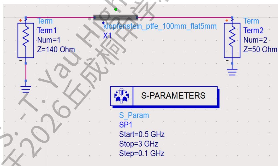
(a) S 参数仿真端口定义
