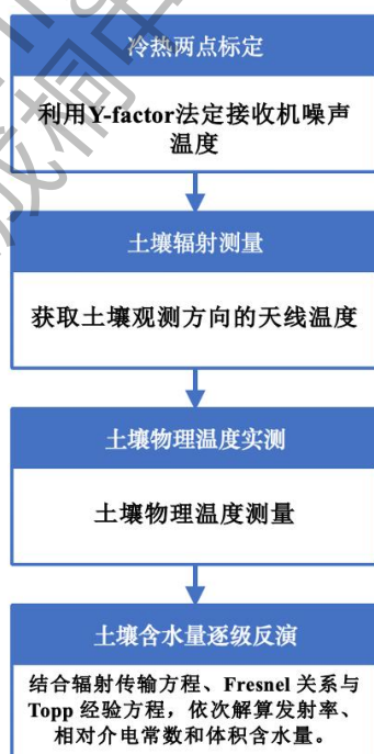
图 4.2 被动式整体逻辑链路
