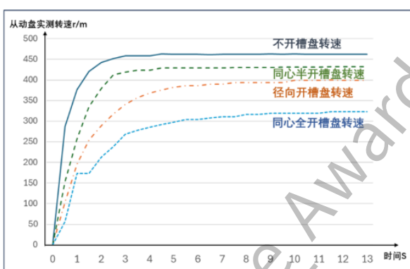
图15 不同形态金属盘转速随时间变化趋势图 (主动盘转速设置: 500r/m)
