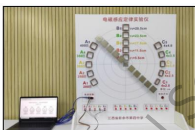
图2(b) 基于Arduino和LabVIEW的电磁感应实验 胡博，中国，2019年
