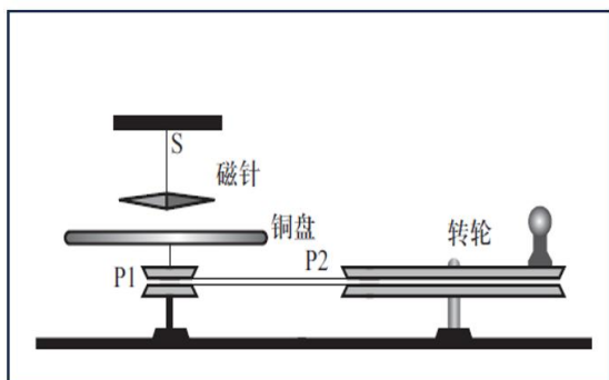
图3(a) 经典阿拉果转盘 Francois Arago, 法国, 1825年
