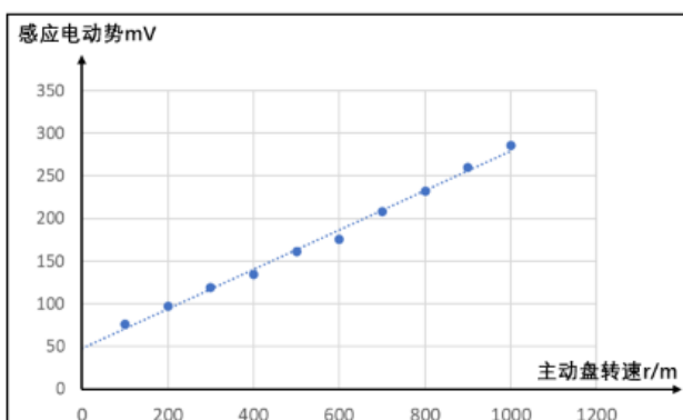
图8 感应电动势趋势图
