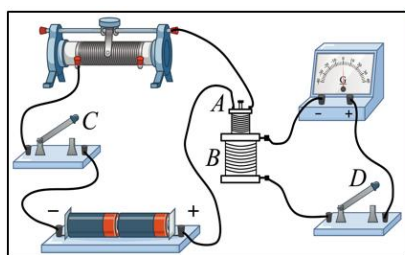
图2(a) 双回路法拉第电磁感应实验 高中物理教材，中国
