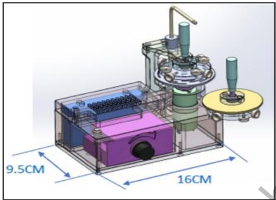
图6 实验装置3D模型 – 主体、支架
