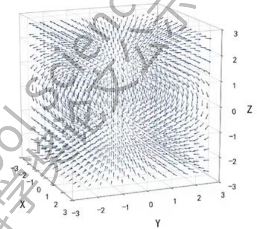
图 4 Python模拟该磁场的三位立体分布图
