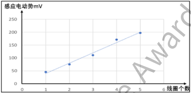
图9 感应电动势趋势图 (主动盘转速设置: 500r/m)
