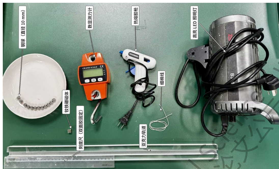
图 2 实验器材。钕铁硼立方磁体（边长 10 mm）、直径 10 mm 的碳钢球、亚克力导轨与沿轨固定的刻度尺；数显测力计用于称量拉脱峰值力，热熔胶枪用于固定磁体，细棉线用于牵引入射球，高亮 LED 照明灯用于保证高速摄影的曝光。
