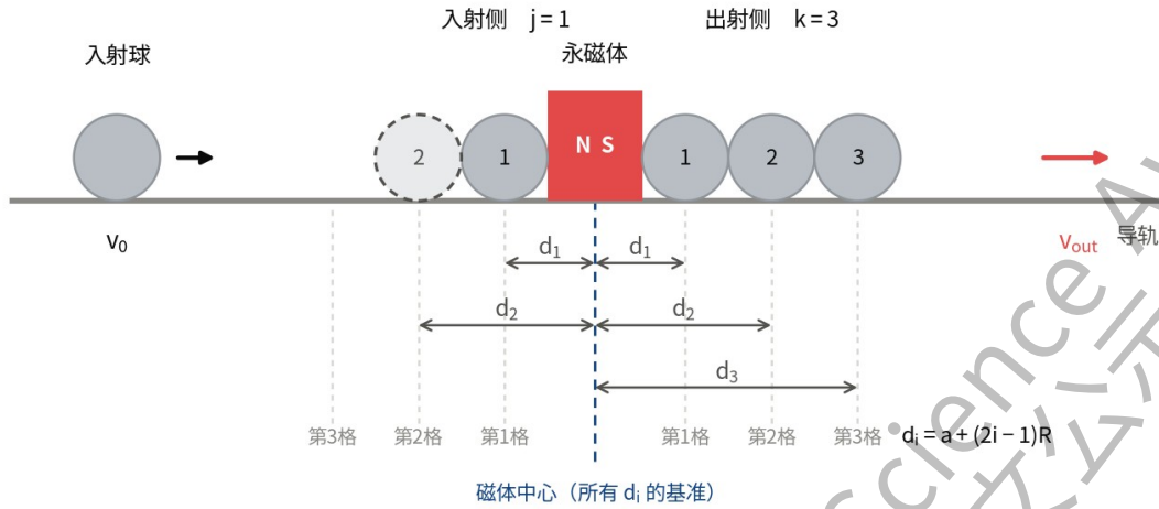
图 1 单组磁力炮的构型。 (j,k) 为待优化的构型参数，图示为 j=1 、 k=3 之一例。虚线圆为入射球被磁体捕获后的最终停靠位置：入射侧第 1 格已被预置球占据，入射球只能停在第 j+1 格。图下方的灰色虚线为格位，各 d_i 均以磁体中心为基准。
