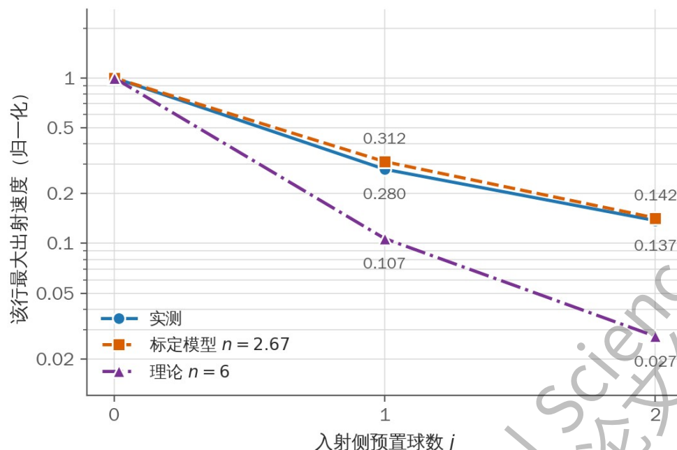
图6 入射侧每多一枚预置球带来的速度损失。纵轴为各行的最大速度，以 j=0 行为1；三条曲线都在测点处求值，与实测同口径。实测的下降幅度（3.6倍、7.3倍）明显小于 n=6 理论的预言（9.4倍、37倍），而与标定后的 n=2.67 模型（3.2倍、7.0倍）接近。
