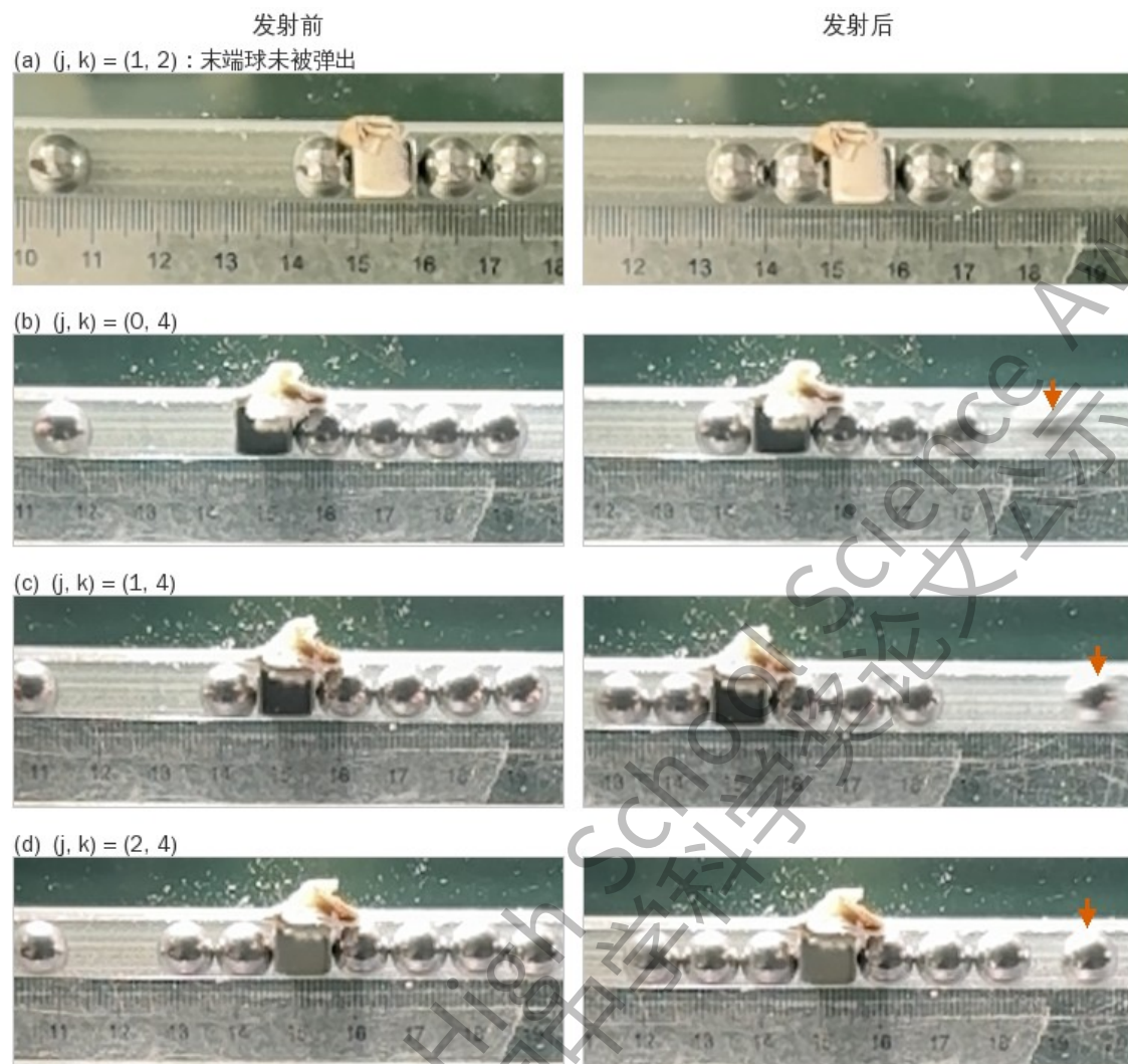
图4 四个构型发射前后的对照。左列为入射球尚在远端时的初始构型，右列为入射球已停靠、末端球已离开之后。(a) (1, 2) 是 k=j+1 的镜像构型，入射球停靠后出射侧球链原样不动；(b)–(d) 的末端球都被弹出，箭头指出它离开球链后的位置，(b)、(c) 中它带有明显的运动模糊。三者的入射球停靠位置随 j 依次由 d_1 后移至 d_2 、 d_3 ，即 2.4 节所指出的、最重要的那一个构型自由度。各分图只作裁切、未作缩放；(a) 摄于另一次装配，胶层较多，摄影比例也比其余三例大约 12%，可由图中的尺子读出。
