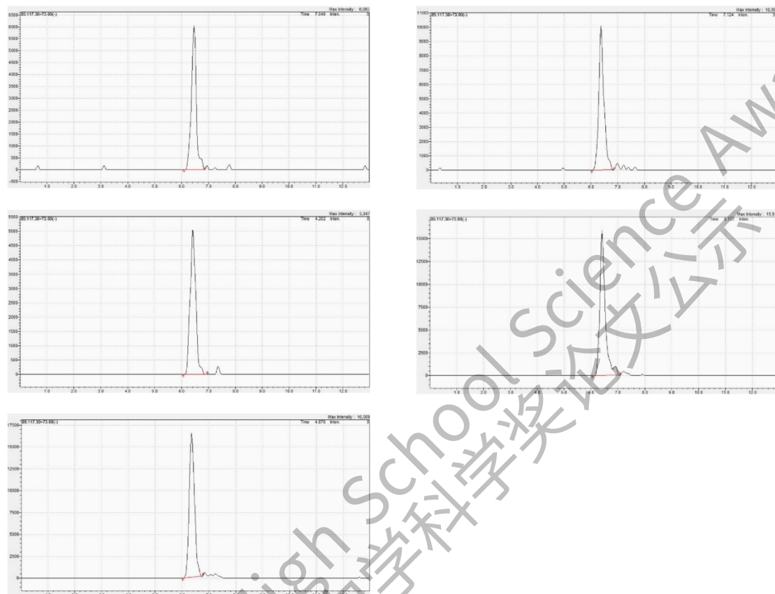
图 S1 LC-MS 提取离子流色谱图分析方法示例。本图横坐标为保留时间，纵坐标为离子丰度。对提取离子流色谱图中具有可识别、基线分离色谱峰的物质进行分析。分析时，目标峰进行积分，得到峰面积。峰面积大小可定性反映相应物质的含量多少。
