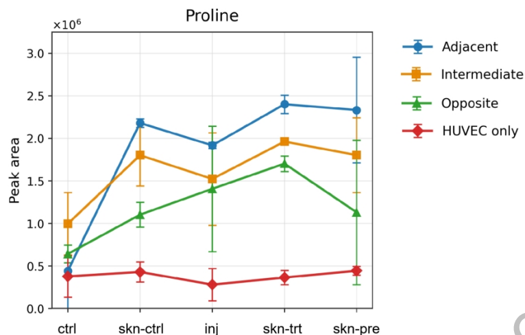
图5 不同处理组中脯氨酸代谢量折线图。
