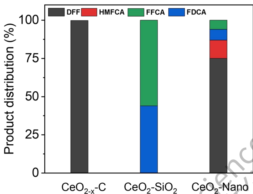
图 3.9 三种氧化铈基催化剂在最大转化率时的产物选择性比较。
