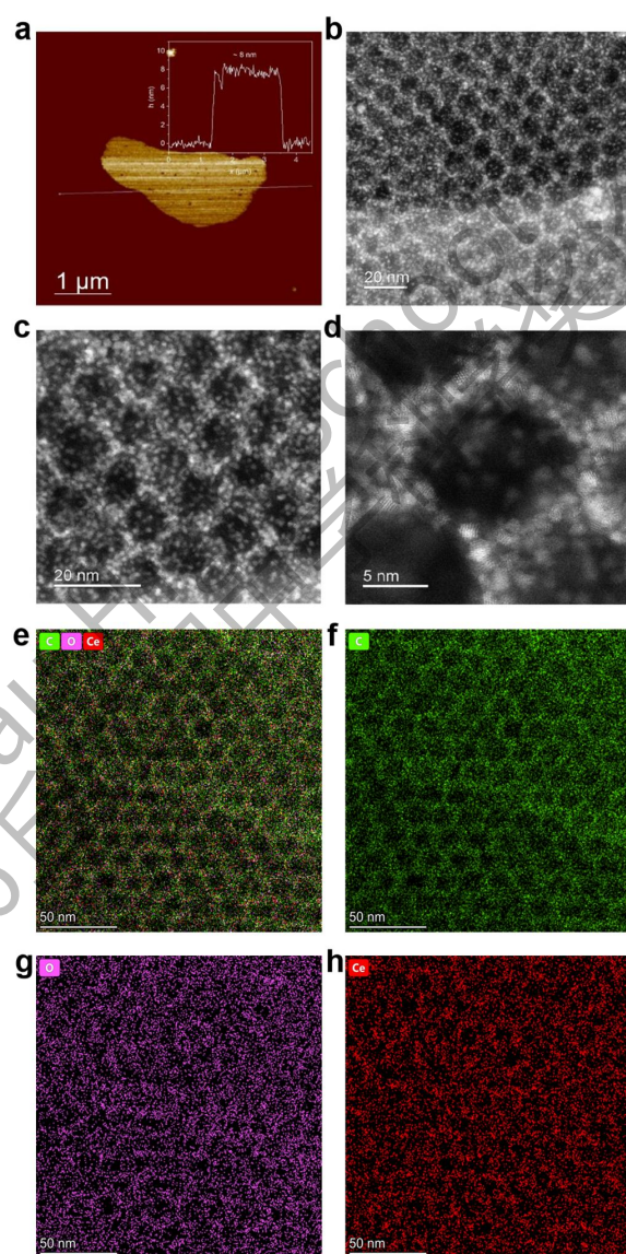
图 3.2 二维介孔 \text{CeO}_{2-x}\text{-C} 纳米片的（a）AFM 图像以及对应沿白线方向的高度曲线；（b-d）不同倍率的 AC-HAADF-STEM 图像；（e-h）图 b 对应的 EDS 元素分布图。
