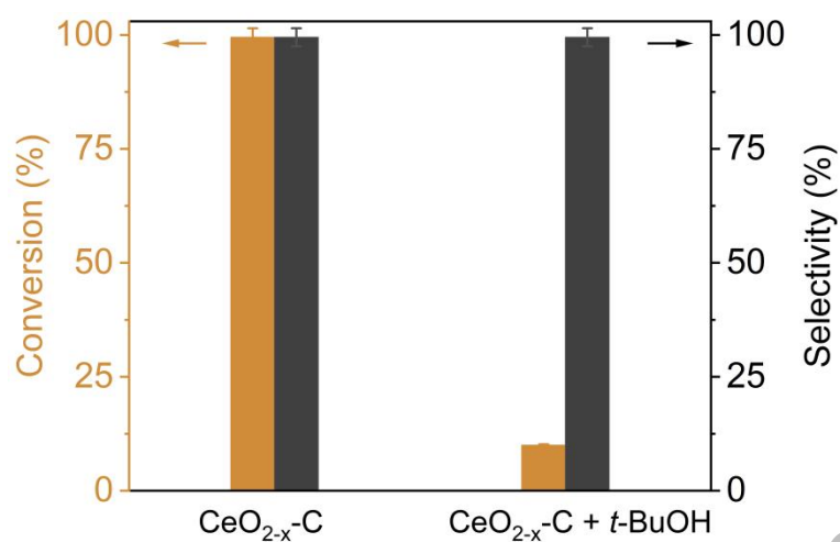
图3.16 叔丁醇 ( t -BuOH) 对HMF转化率和DFF选择性的影响。
