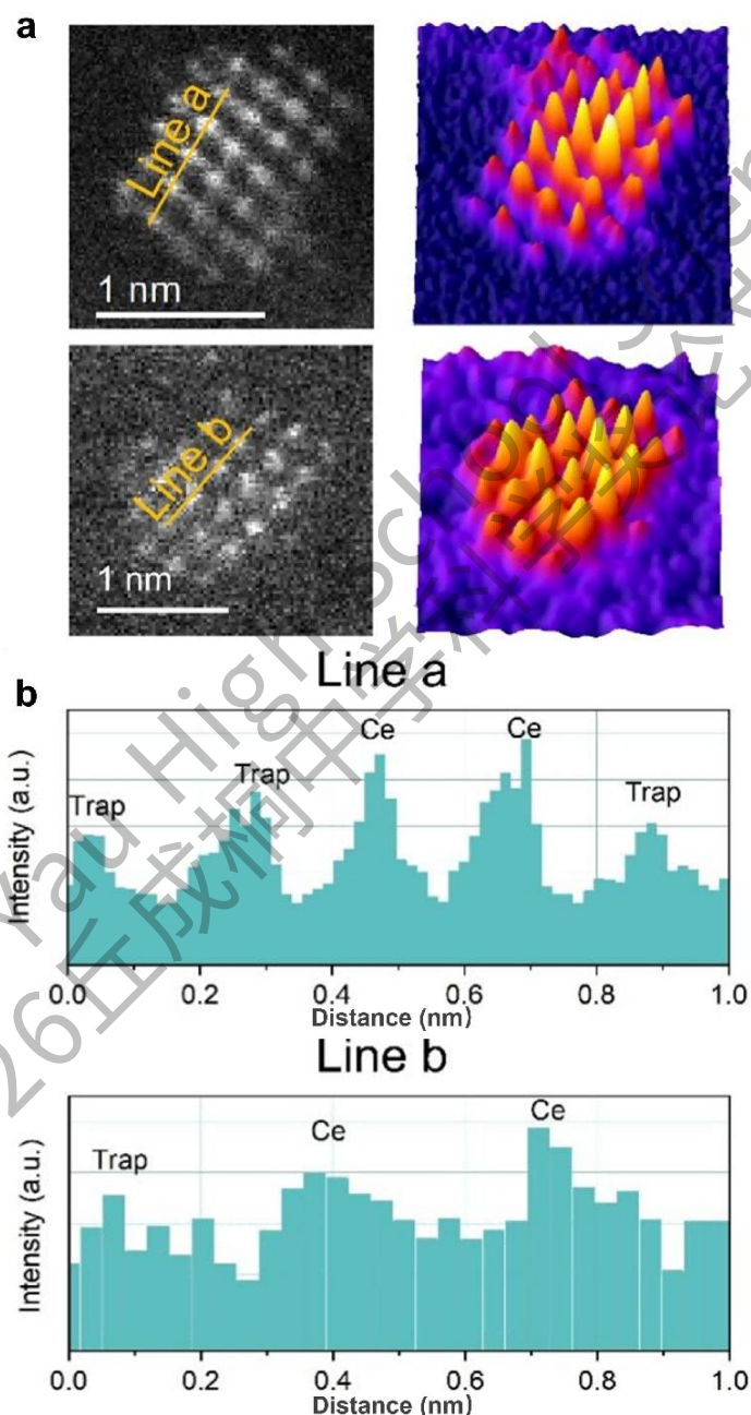
图 3.3 二维介孔 CeO 2-x -C 纳米片中（a）典型 CeO 2-x 团簇的 AC-HAADF-STEM 图像及对应的三维转化图；（b）沿图 a 中提取线的强度剖面。
