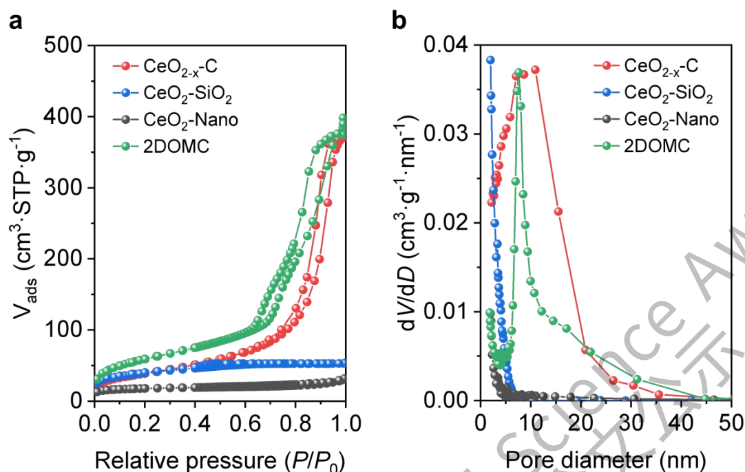
图 3.7 三种 \text{CeO}_2 基样品以及二维介孔碳纳米片 2DOMC 的 (a) \text{N}_2 吸附-脱附等温线和 (b) 孔径分布图。
