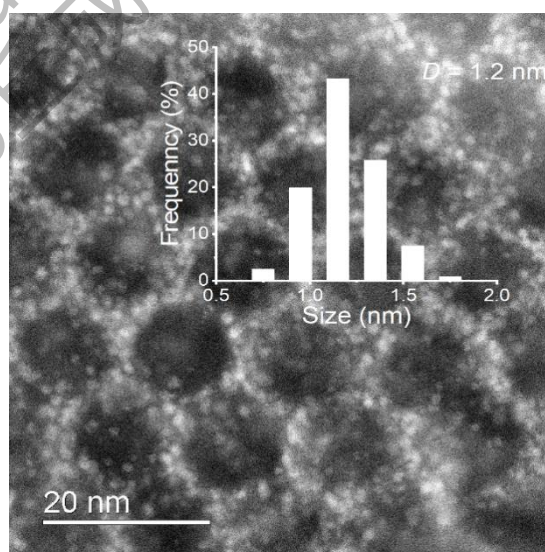
图3.12 循环使用10次后 \text{CeO}_{2-x}\text{-C-R} 催化剂的AC-HAADF-STEM像。
