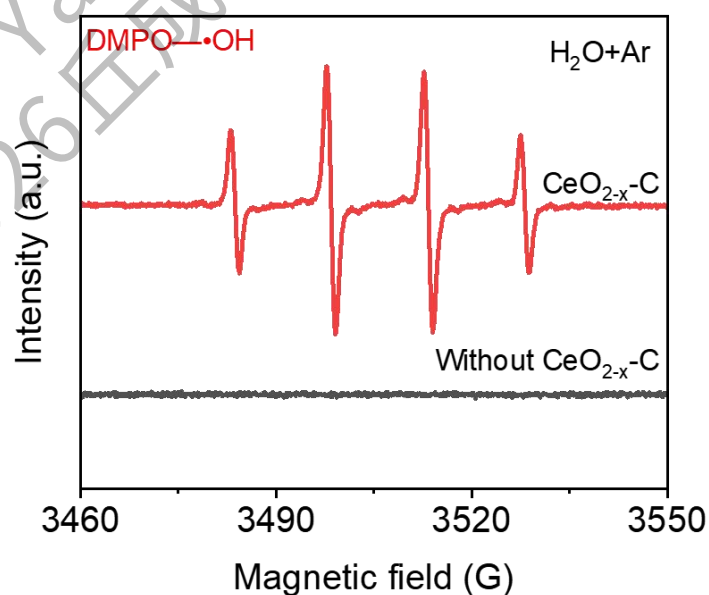
图3.15 二维介孔CeO 2-x -C催化HMF氧化DMPO捕获ESR谱图。
