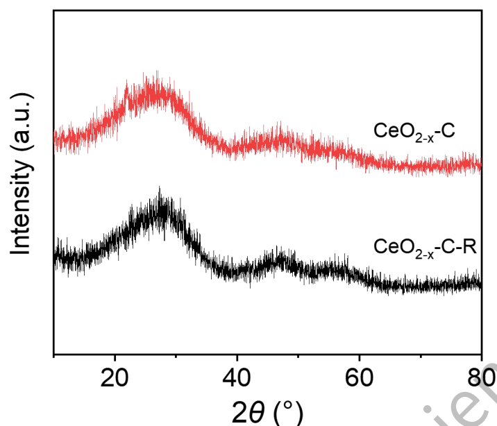
图3.13 新鲜 \text{CeO}_{2-x}\text{-C} 催化剂和循环反应后催化剂（ \text{CeO}_{2-x}\text{-C-R} ）的XRD谱图。
