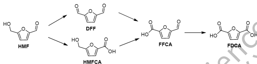
图 1.2 HMF 氧化/脱氢反应网络。
