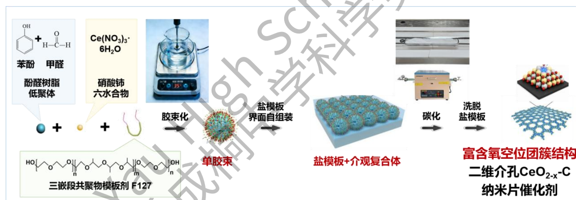
图 3.1 二维介孔 \text{CeO}_{2-x}\text{-C} 纳米片的合成流程示意图。
