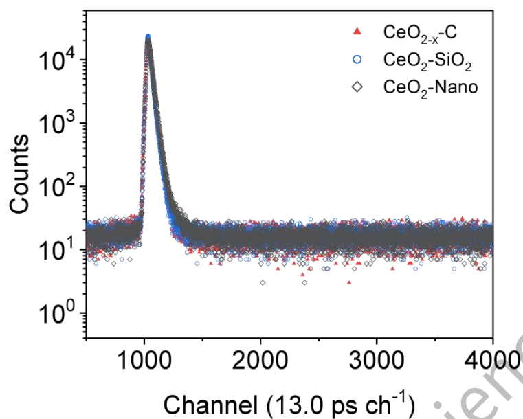
图3.6 \text{CeO}_{2-x}\text{-C} 、 \text{CeO}_2\text{-SiO}_2 与 \text{CeO}_2\text{-Nano} 样品的正电子湮没寿命谱。
