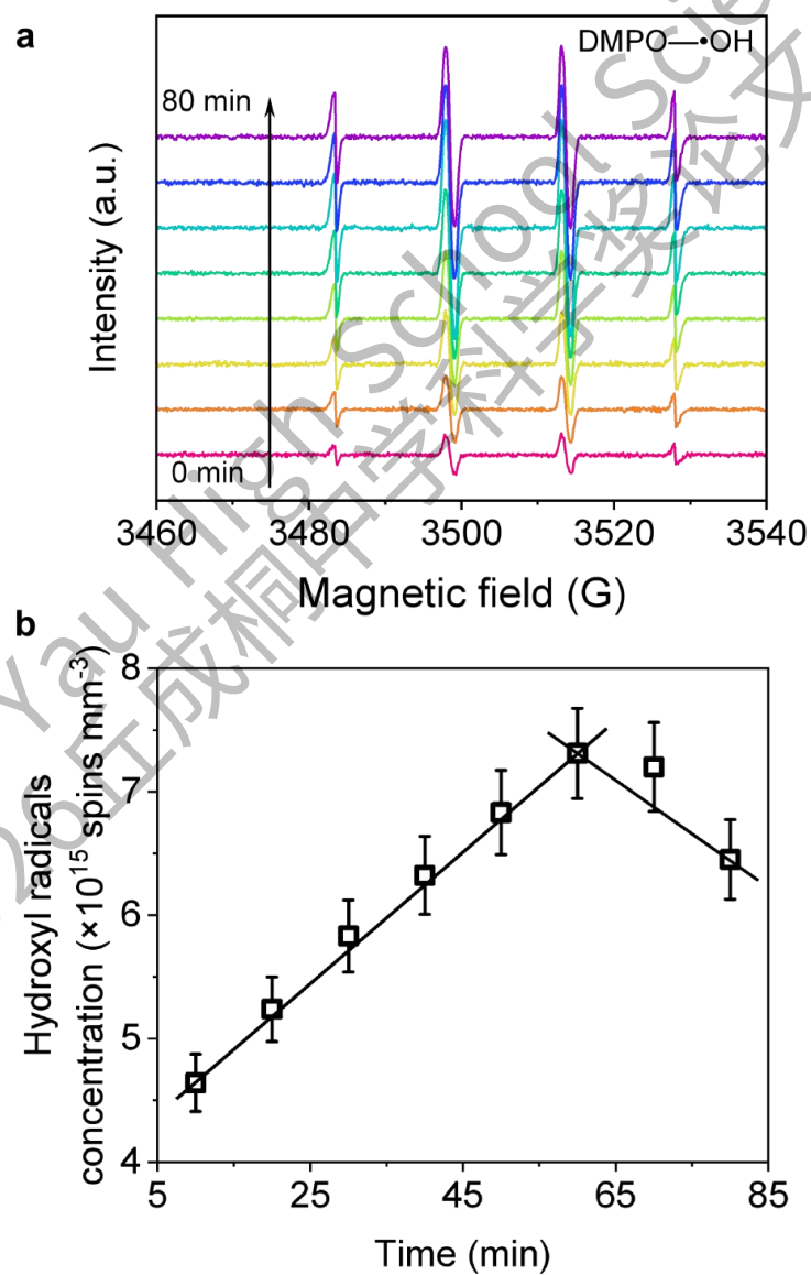
图 3.17 (a) DMPO·OH 信号随反应时间的变化及 (b) 其表观浓度。
