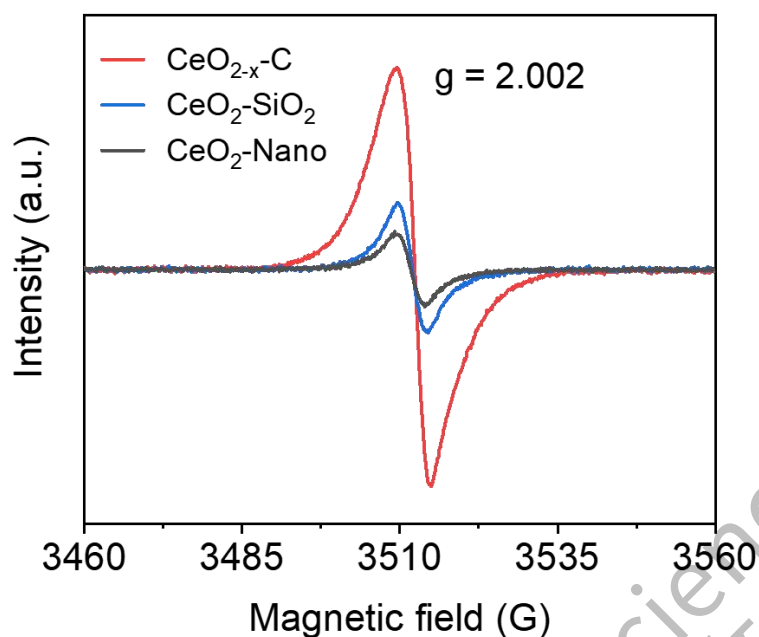
图3.5 \text{CeO}_{2-x}\text{-C} 、 \text{CeO}_2\text{-SiO}_2 与 \text{CeO}_2\text{-Nano} 样品的ESR谱。
