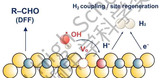
图 3.20 富含氧空位 \text{CeO}_{2-x} 团簇仅以水参与 HMF 氧化脱氢的反应路径示意图。
