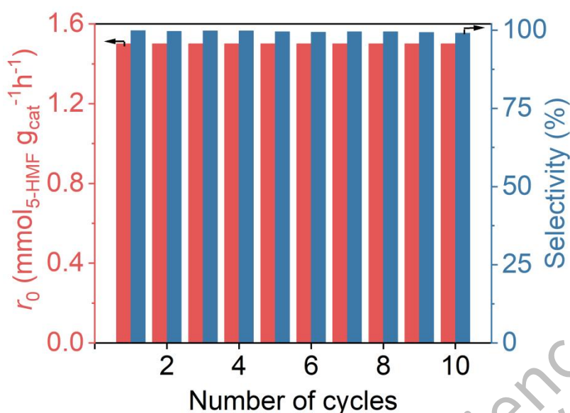
图3.11 催化剂循环稳定性结果。
