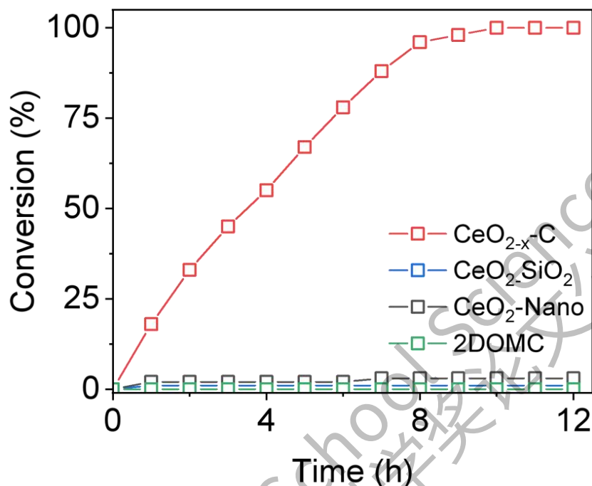
图 3.8 不同催化剂上 HMF 转化率随时间的变化曲线。
