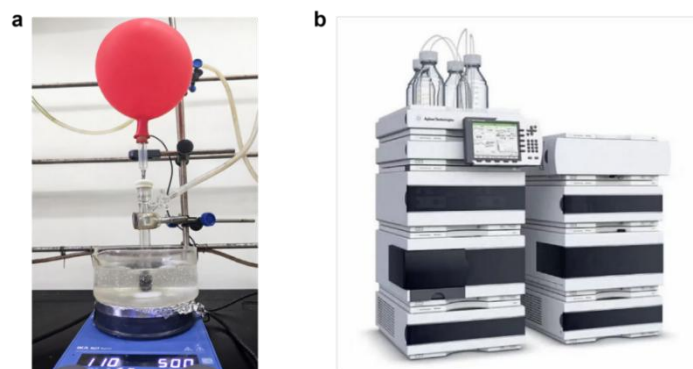
图 2.1 (a) 催化反应装置和 (b) 高效液相色谱。
